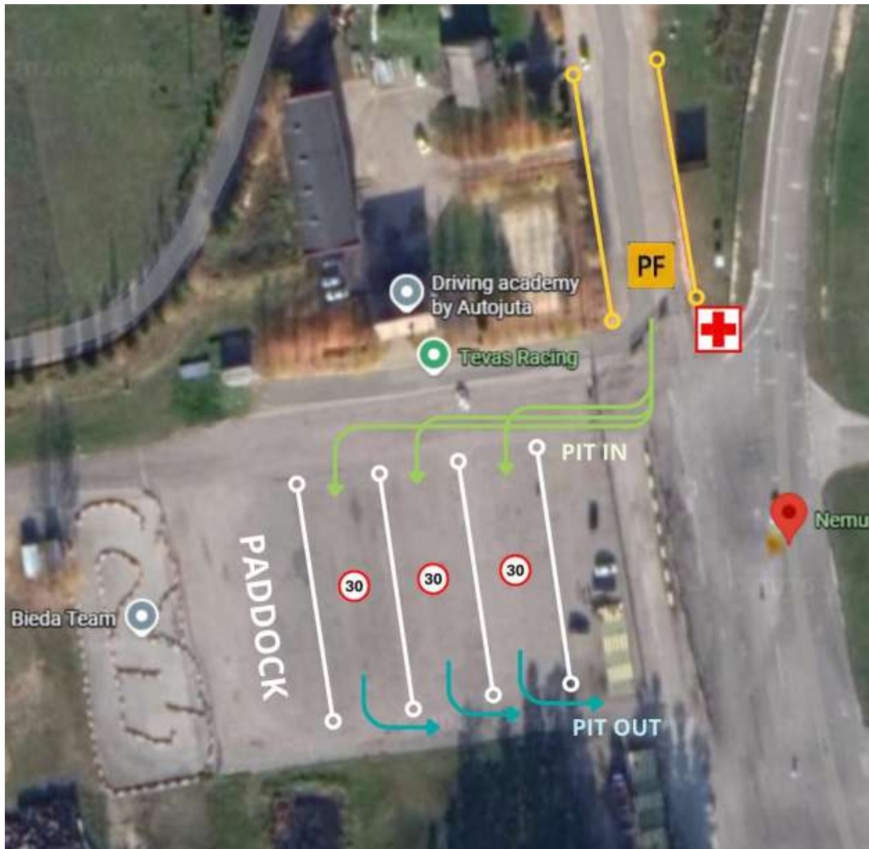
Paddock ir Pit lane schema
